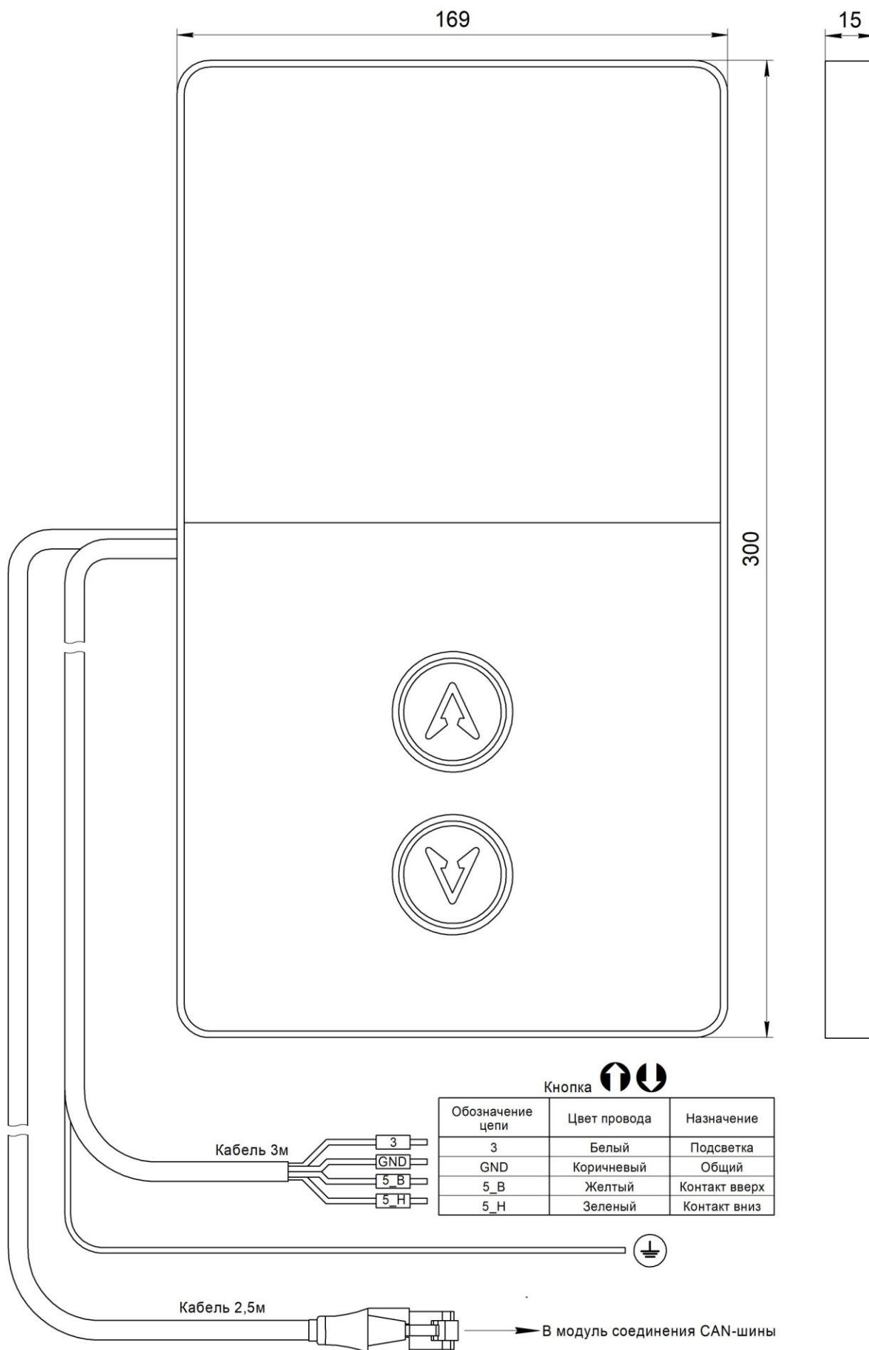
Рис.1 Внешний вид Вызывной пост ОНИКС (жгут RJ45) НШЕК.468381.024
